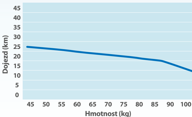
Dojezd (km) v závislosti na hmotnosti (kg)
