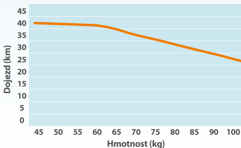
Dojezd (km) v závislosti na hmotnosti (kg)
